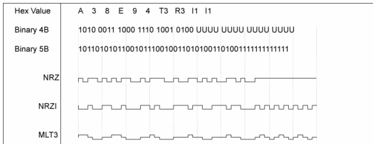
Figure 20. MLT3 Coding
